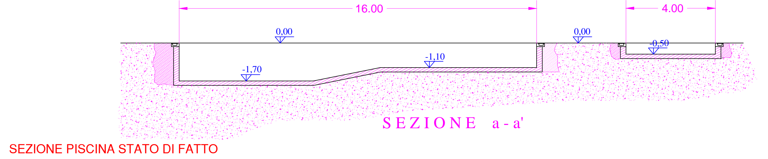
SEZIONE PISCINA STATO DI FATTO
