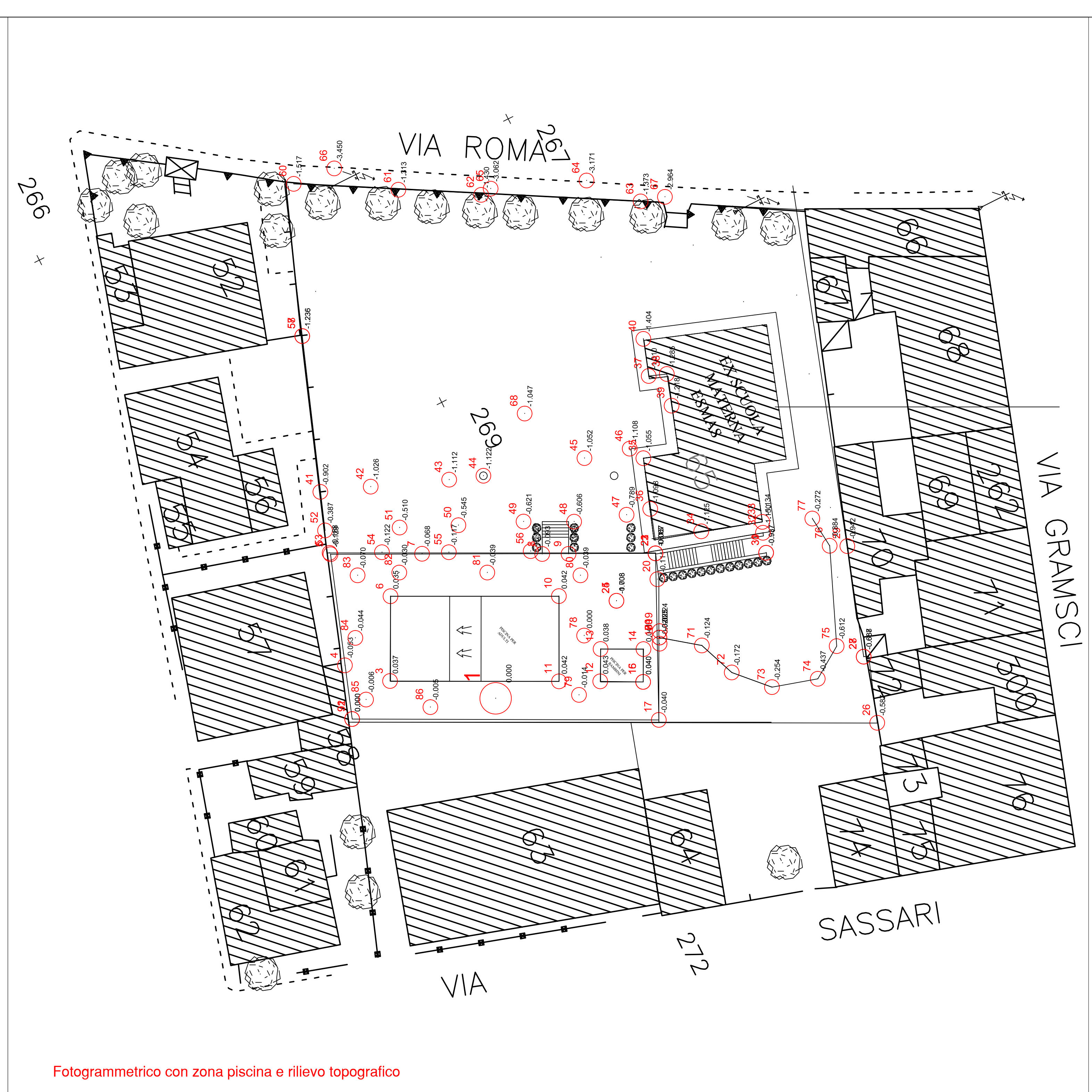
Fotogrammetrico con zona piscina e rilievo topografico
